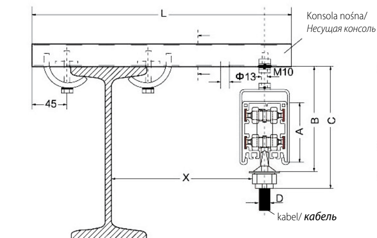
Konsola nośna Zacisk dla D=6–15 mm / Несущая консоль Зажим для D=6–15 mm
